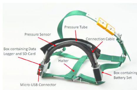
Figura 3. Sistema de monitoramento da alimentação - RumiWatch ® [9].
