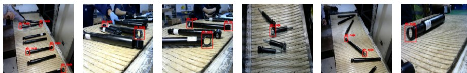
Fig 1: Detección automática de faltante de bujes en línea de producción de amortiguadores.
