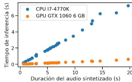
Fig. 1. Tiempo de síntesis del sistema respecto a la duración del audio sintetizado. Se muestran los resultados obtenidos en un mismo equipo, cambiando solamente el hardware en el que se realiza la inferencia (CPU vs GPU).
