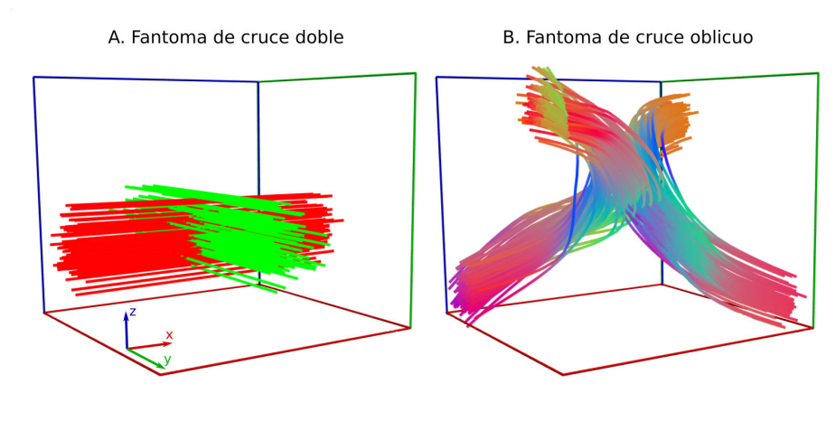
Figura 2. Disposición de las fibras en los fantomas diseñados para probar el modelo propuesto. A) En rojo la fibra en dirección x del primer fantoma, en combinación con la fibra en dirección y en verde (segundo fantoma). B) Las dos fibras curvadas que se cruzan, del tercer fantoma.
